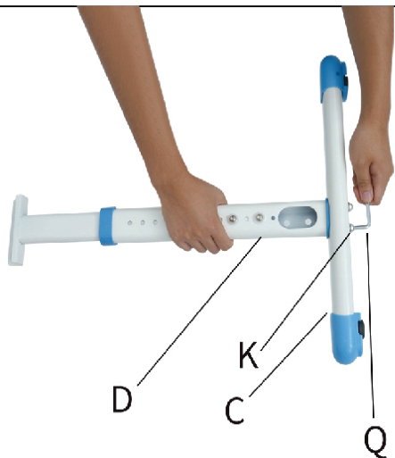
Шаг 1. Соберите ногу каркаса
