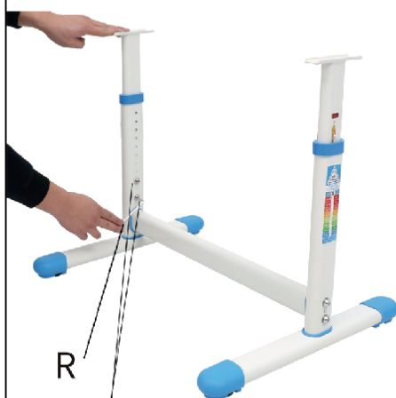
Шаг 5. Ослабьте винты и настройте опору под высоту стула
