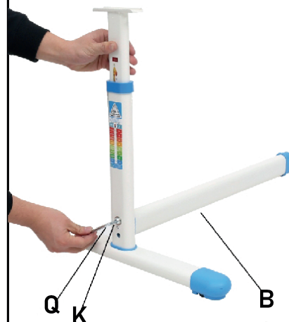
Шаг 3. Присоедините опору
